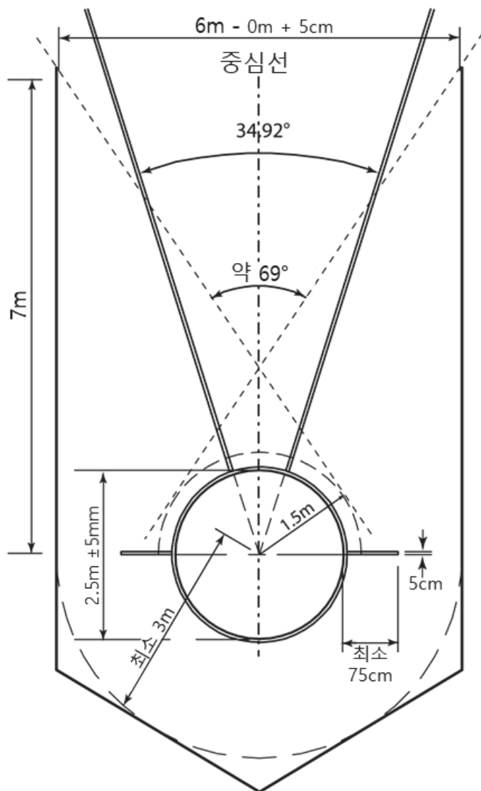
그림 TR35 원반던지기 전용 그물장의 설계도
