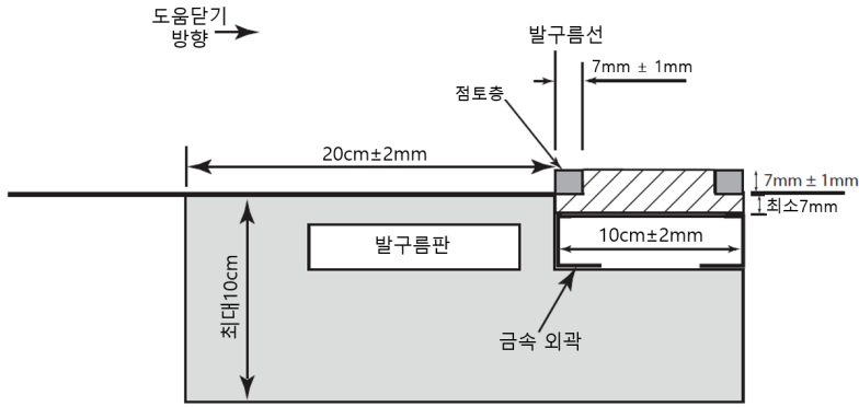
그림(a2) TR29 발구름판과 점토판
