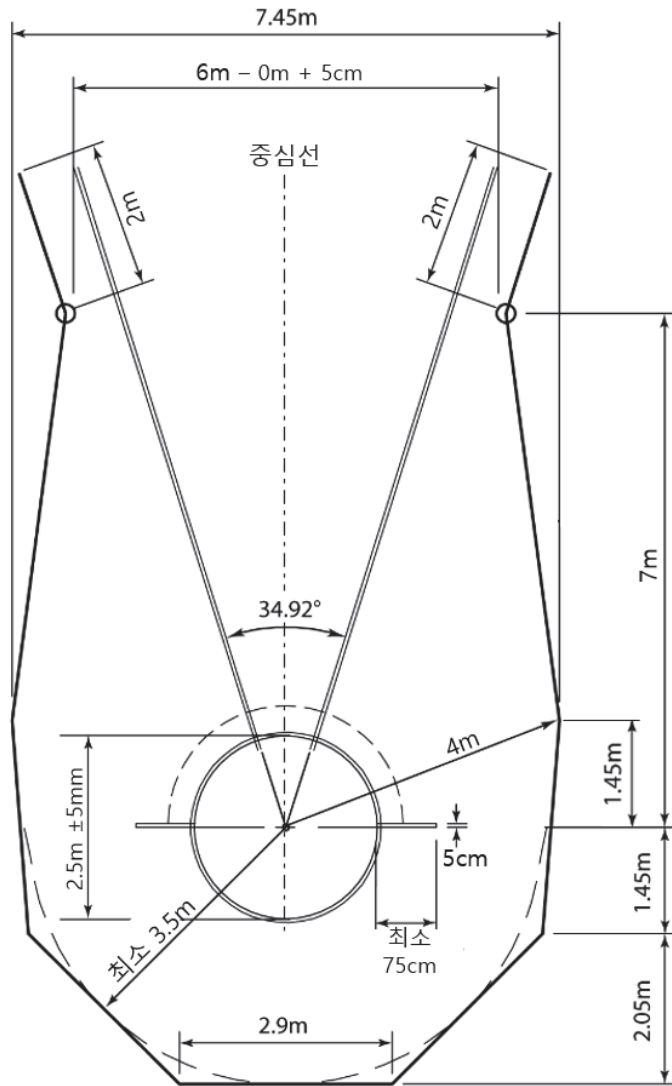
그림(b) TR37 동심원서클의 해머 및 원반던지기 그물장 (원반던지기 배치 및 그물망에 대한 그물장 치수)
