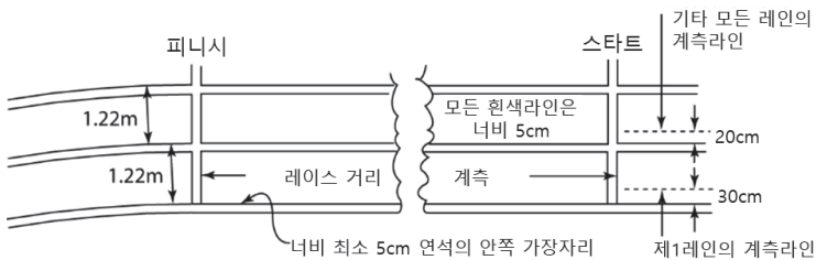
그림 TR14 트랙 계측(필드 내에서 본 도안)
