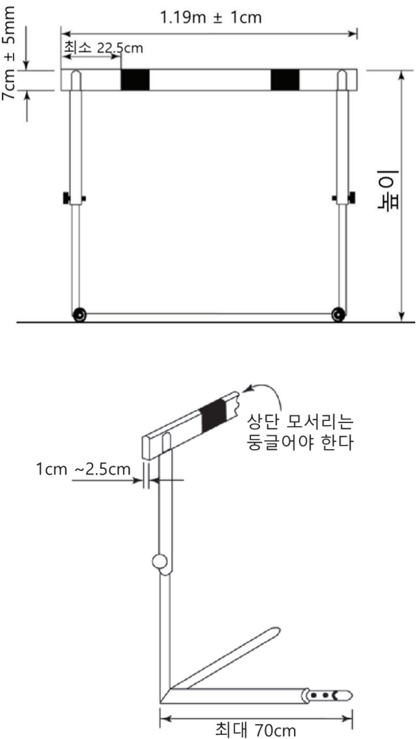
그림 TR22 허들 (예)
