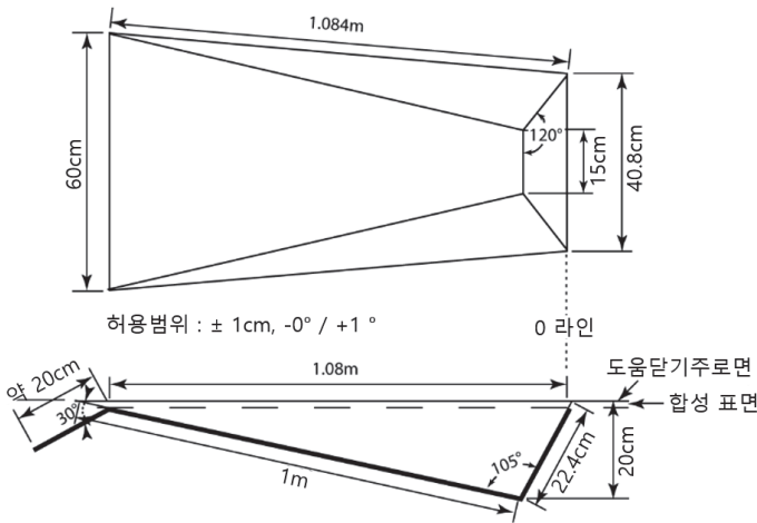
그림(a) TR28 장대높이뛰기 박스(상단 및 측면에서 본 그림)
