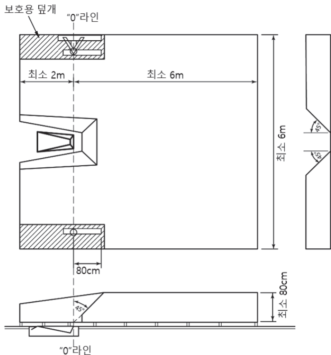
그림(c) TR28 장대높이뛰기 착지장소(상단 및 측면에서 본 그림)
