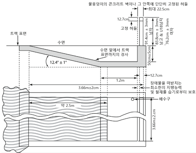
그림(b) TR23 물웅덩이 (Water jump)
