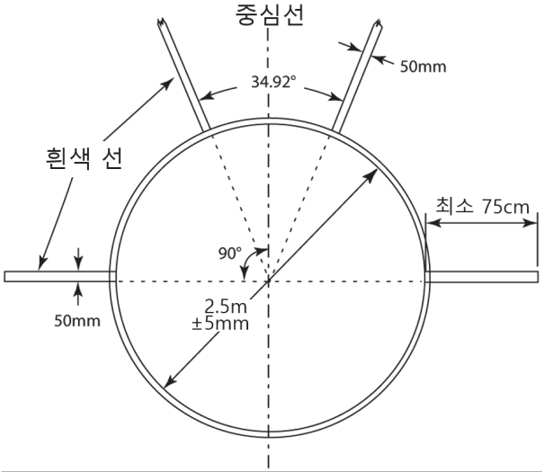
그림(b) TR32 원반던지기서클 설계도
