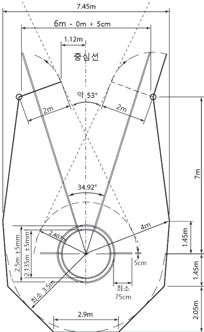
그림(a) TR37 동심원서클의 해머 및 원반던지기 그물장 (오른손잡이 선수용 해머던지기 배치 및 그물망에 대한 그물장 치수)
