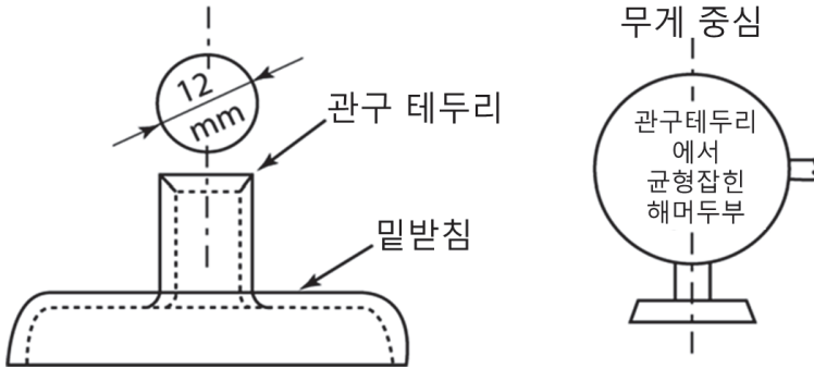
그림(a) TR36 해머두부 무게중심 검사기구
