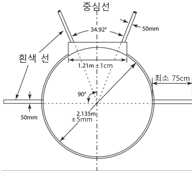
그림(a) TR32 포환던지기서클 설계도
