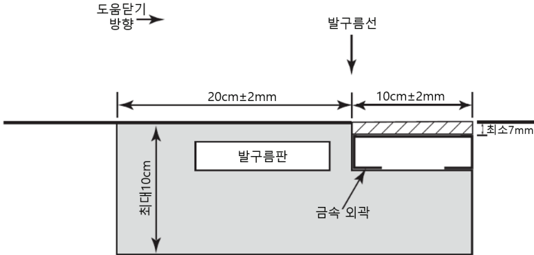
그림(a1) TR29 발구름판과 평탄한 점토판
