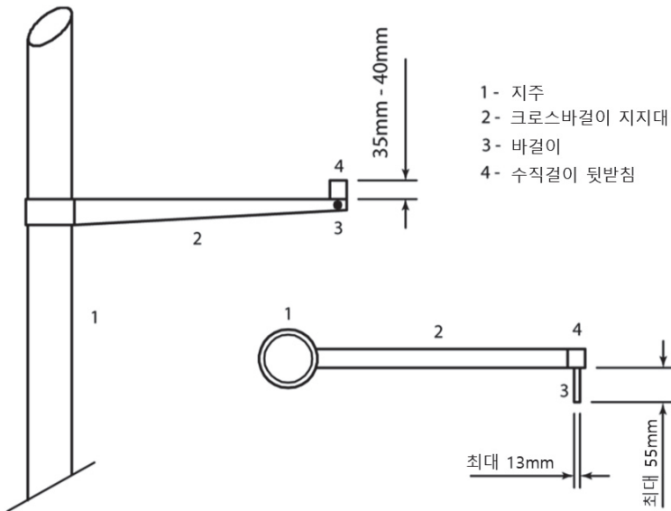
그림(b) TR28 장대높이뛰기 크로스바결이 지지대(착지장소 및 위에서 본 그림)
