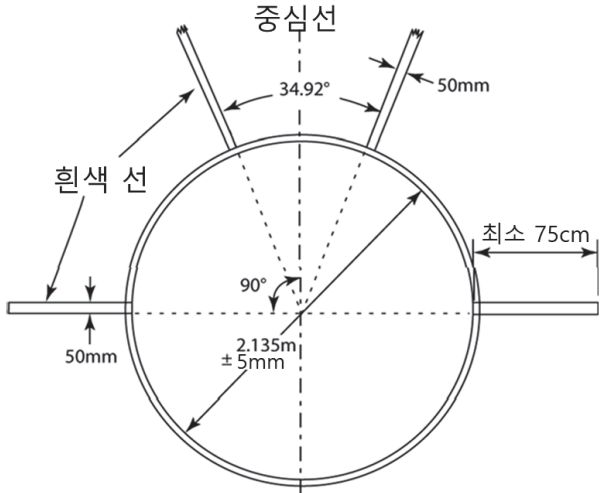
그림(c) TR32 해머던지기서클 설계도
