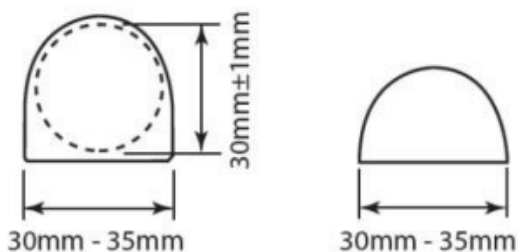
그림 TR26 크로스바 끝부분의 대체 형태
