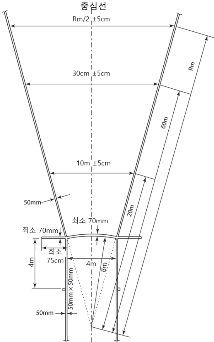
그림(e) TR32 창던지기 도움달기주와 낙하구역
