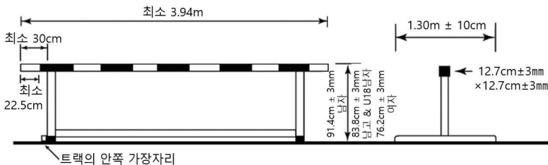
그림 (a) TR23 장애물 허들(예)
