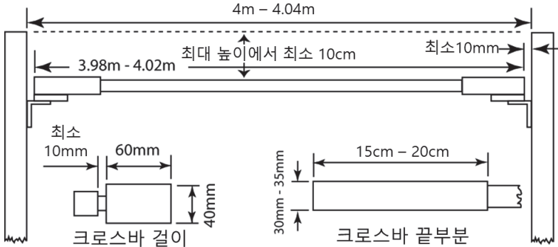
그림 TR27 높이뛰기 지주와 크로스바
