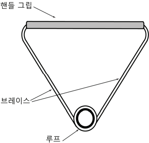
그림(b) TR36 일반적인 해머 핸들
