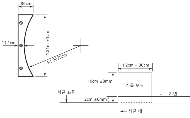
그림 TR33 포환던지기 스톱보드(상단 및 측면에서 본 모습)
